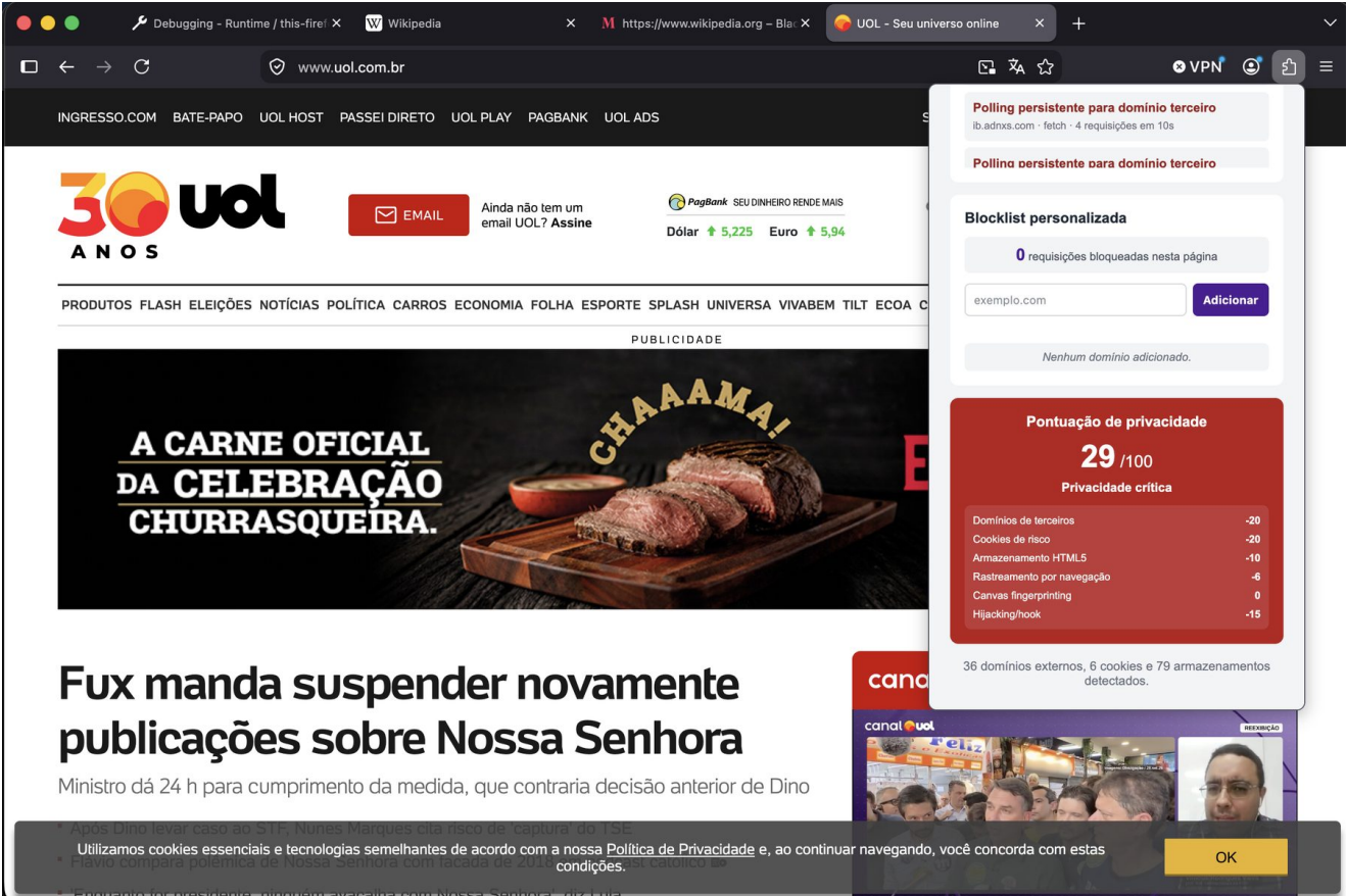
Figura 25 - UOL: pontuação e blocklist.
