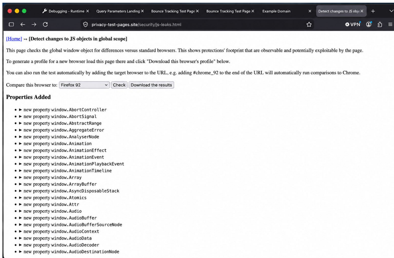
Figura 15 - JS Leaks: resultado da comparação de superfície.
