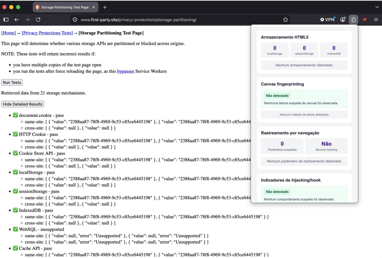
Figura 9 - Storage Partitioning: top document sem chaves enumeradas.
