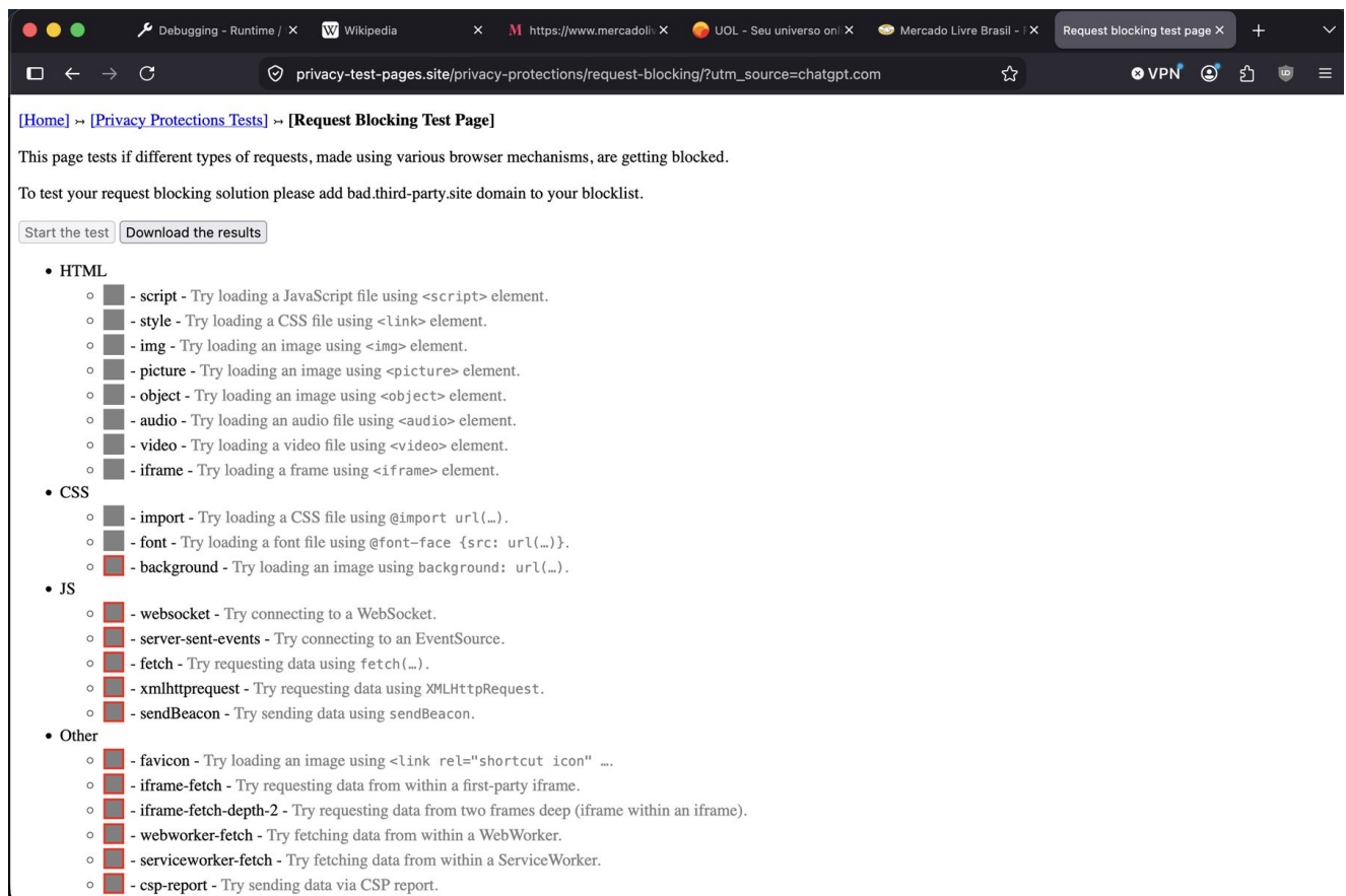
Figura 4 - Tracker Blocking: resultados reportados pela página.
