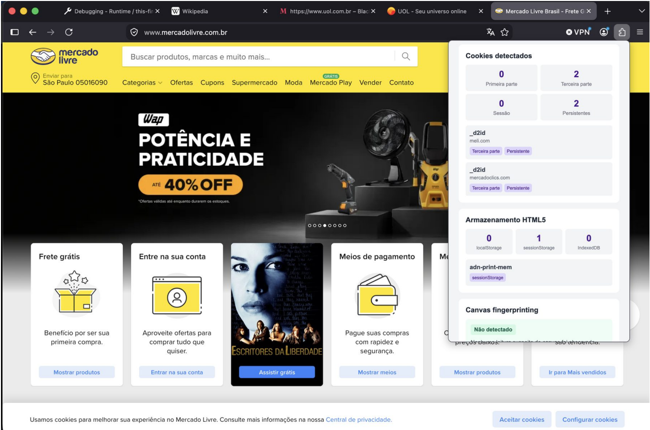
Figura 29 - Mercado Livre: cookies e armazenamento.
