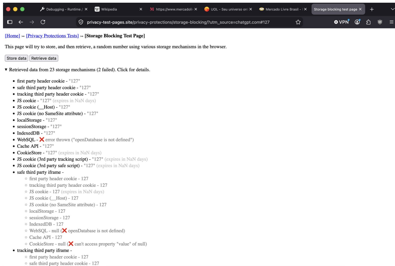
Figura 6 - Storage Blocking: resultados da página.
