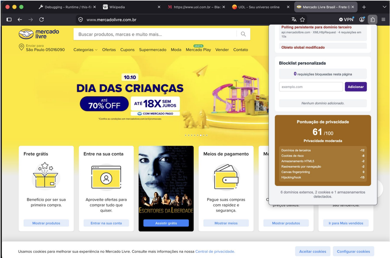
Figura 31 - Mercado Livre: pontuação e blocklist.
