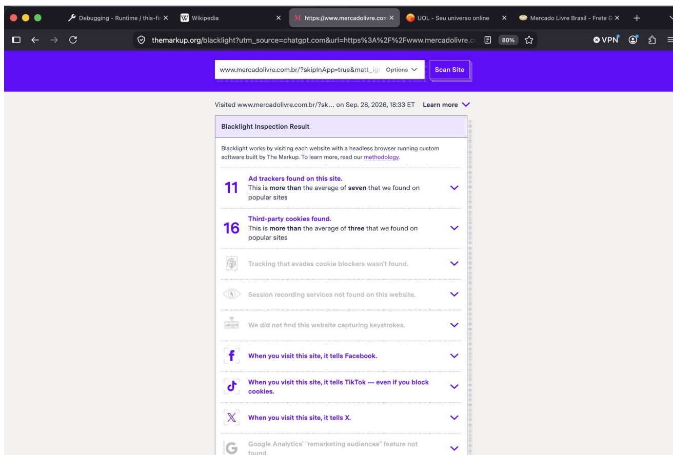
Figura 32 - Mercado Livre: resultado do Blacklight.
